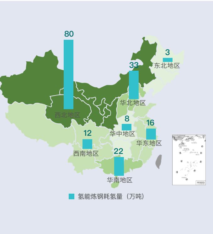
图表 23 2030年中国氢能炼钢耗氢量分布
